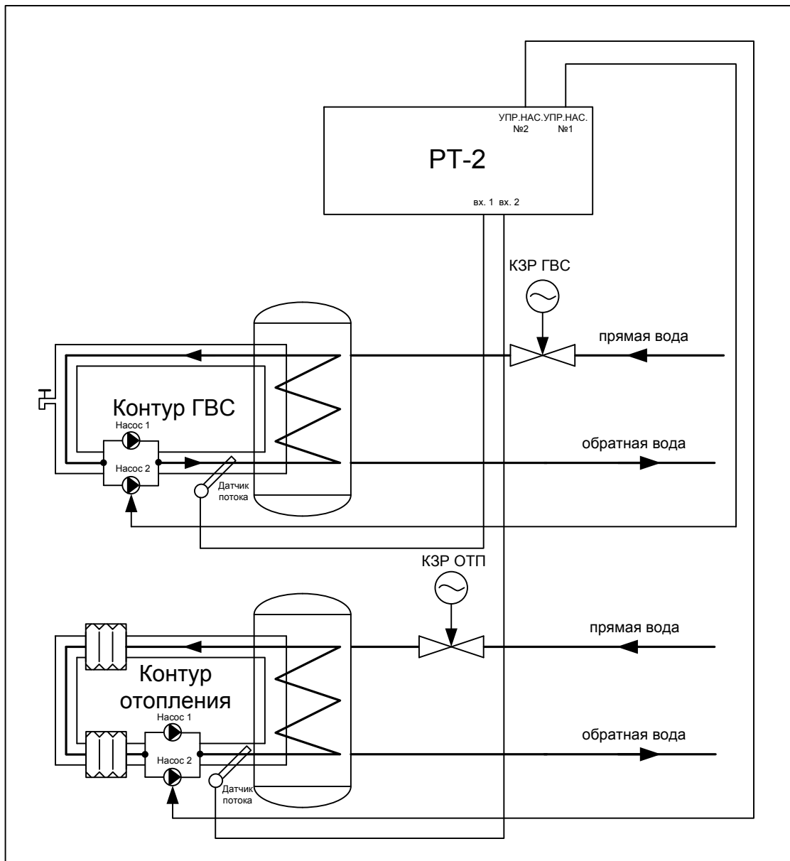
Рисунок П 2.1. Схема подключения регулятора РТ-2 при использовании на ЦТП (ИТП) для управления работой насосов.
