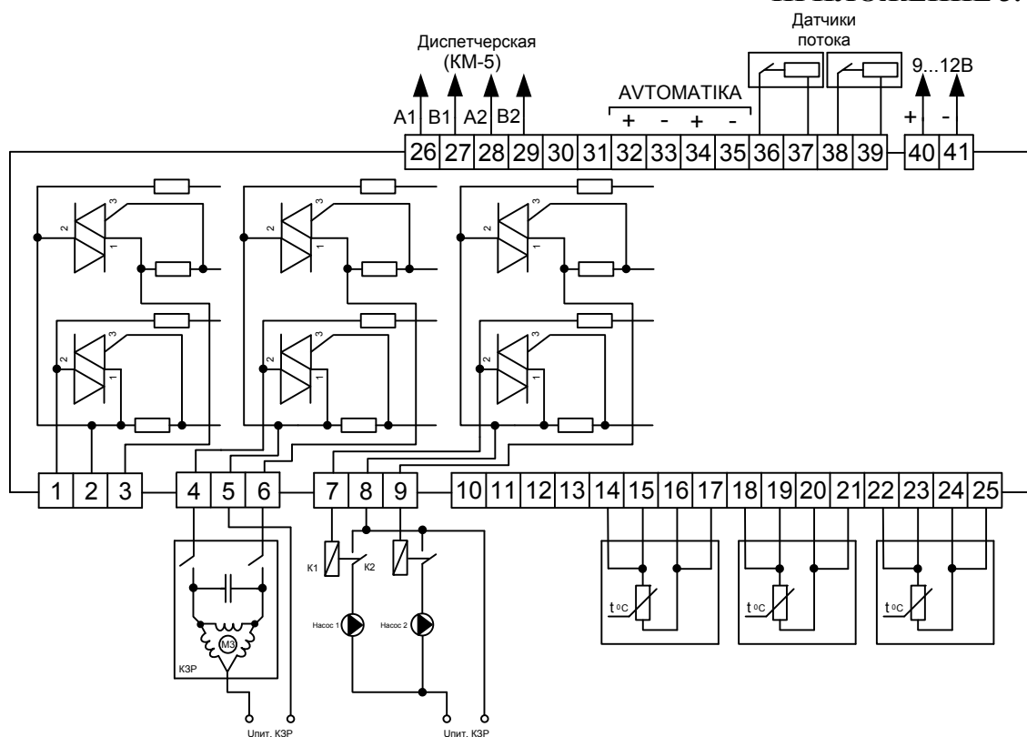
Рисунок П 3.4. Электрическая схема подключения (для гидравлических схем, приведенных на Рисунках П3.1. и П 3.2.)
