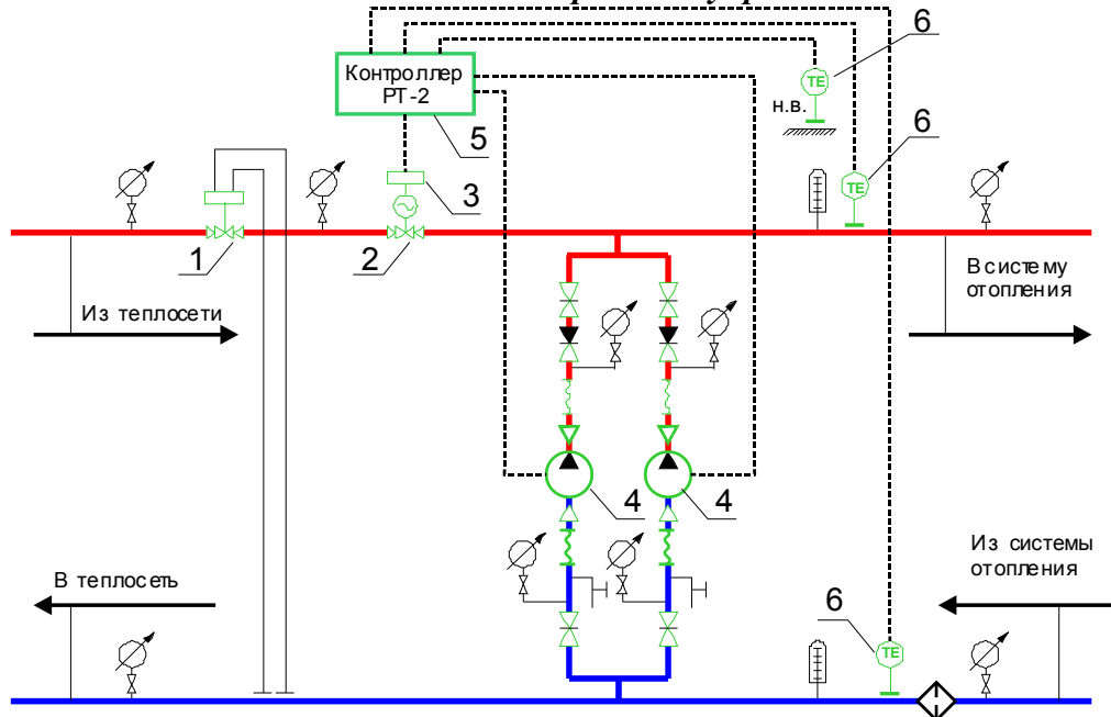
Рисунок П 3.1. Принципиальная гидравлическая схема подключения с насосами на перемычке.
