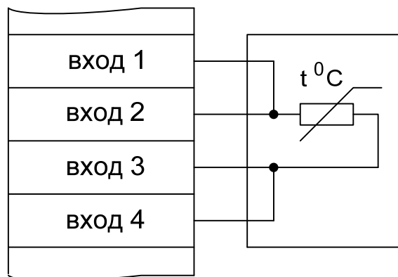
Рисунок П 4.2. Электрическая схема подключения термометров сопротивления.
