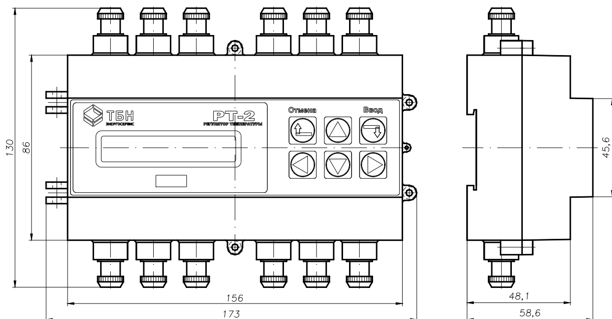
Рисунок 1с. РТ-2 в моноблочном исполнении.
