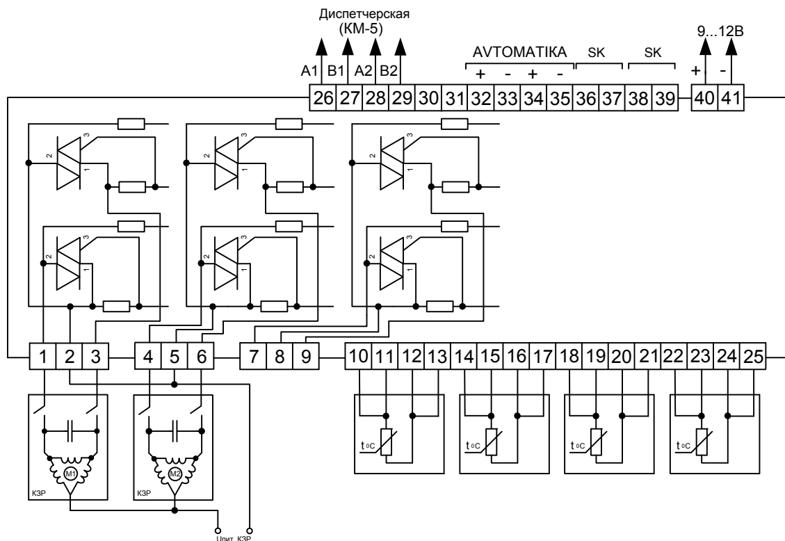
Рисунок П 3.9. Электрическая схема подключения (для схемы подключения регулятора РТ-2, приведенной на Рисунке П3.8 ).
