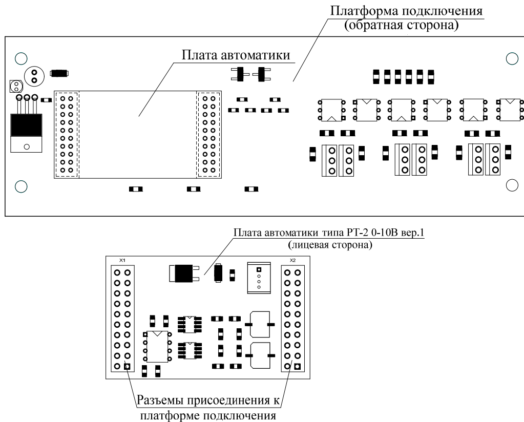
Рисунок 1а. РТ-2 в раздельном исполнении в шкафу производства ООО «ТБН энерго-сервис».
