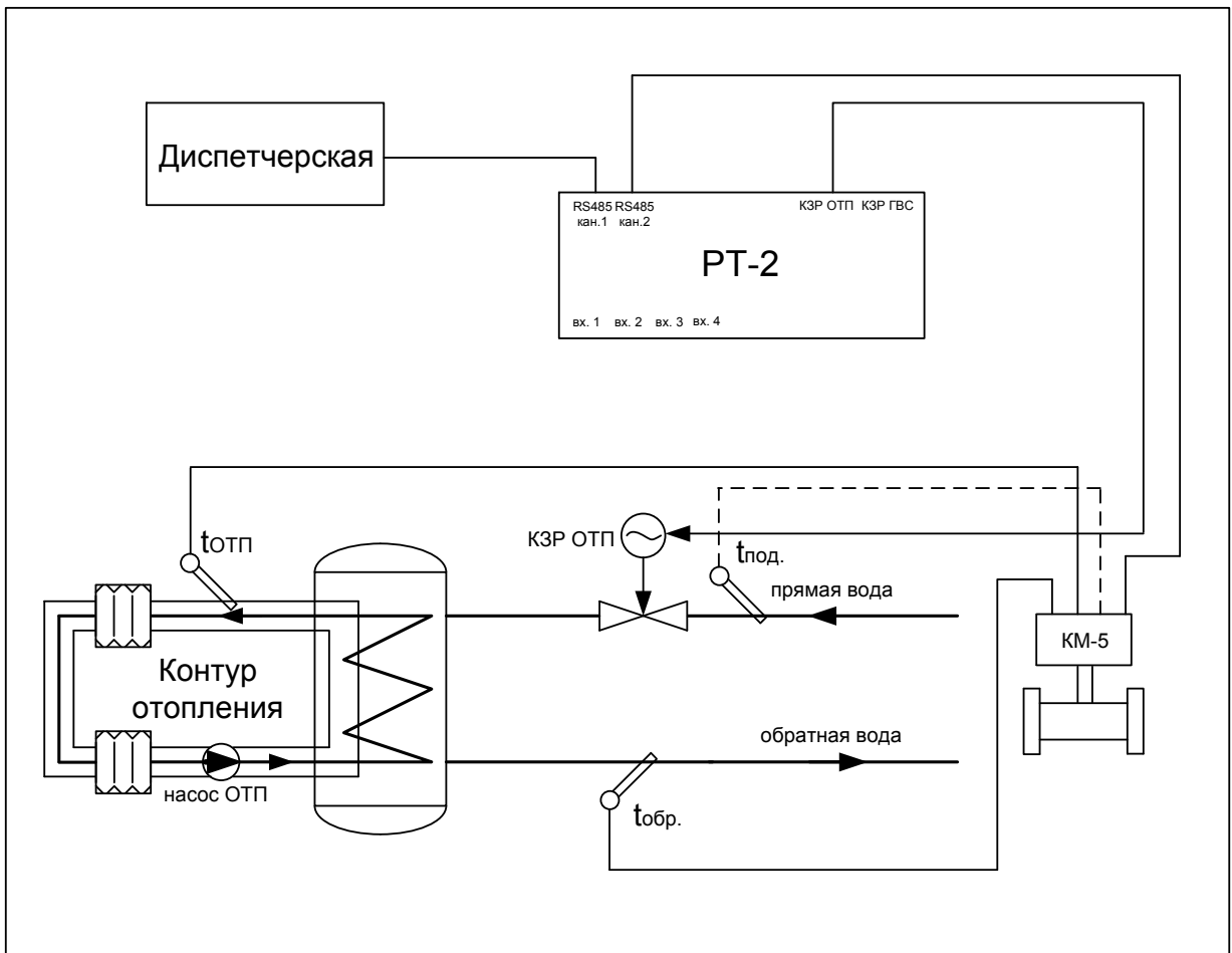
Рисунок П 2.2. Схема подключения регулятора РТ-2 на узле регулирования и учета при совместном использовании с теплосчетчиком КМ-5 .
