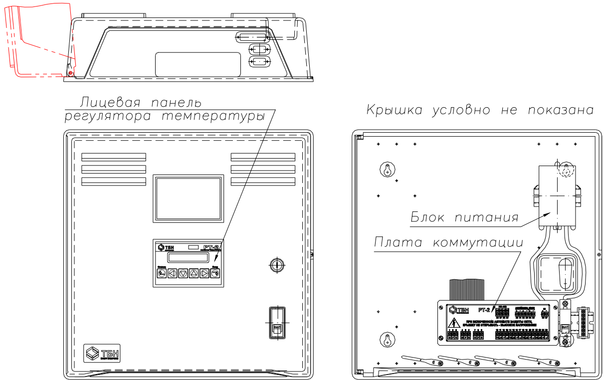
Рисунок 1а. РТ-2 в раздельном исполнении в шкафу производства ООО «ТБН энерго-сервис».
