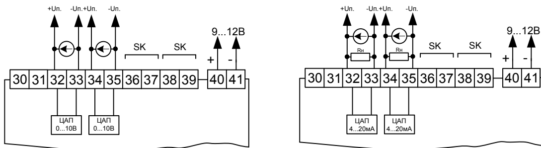
Рисунок П 1.3. Схема подключения исполнительных механизмов с управлением напряжением 0 ... 10 В и током 4... 20 мА к выходам ЦАП регулятора РТ-2.
