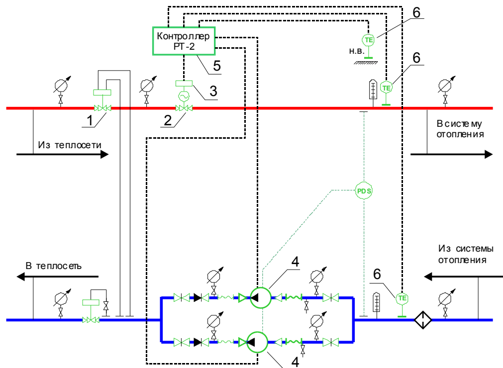
Рисунок П 3.2. Принципиальная гидравлическая схема подключения с насосами на обратном трубопроводе.
