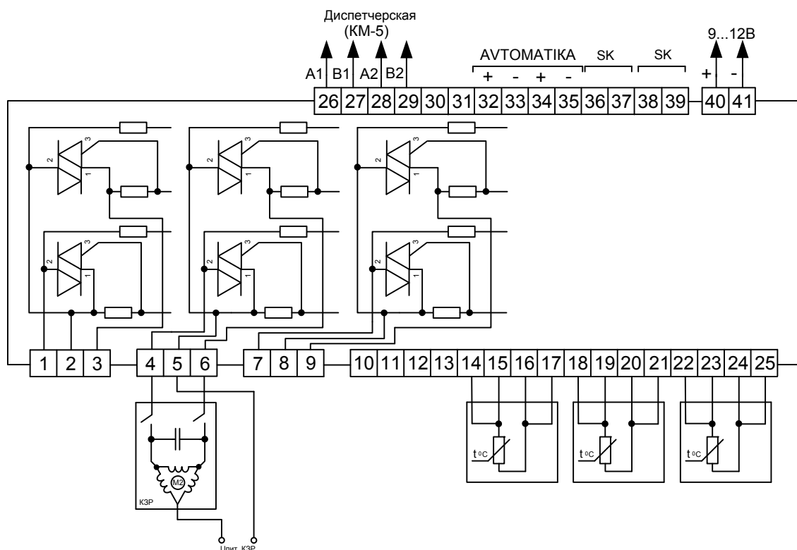
Рисунок П 3.6. Электрическая схема подключения (для гидравлической схемы, приведенной на Рисунке П3.5 ).
