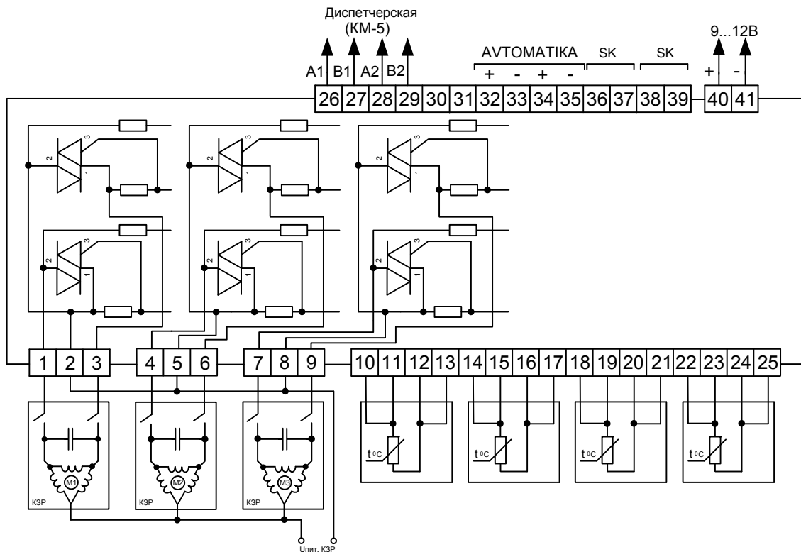
Рисунок П 1.1. Схема электрических подключений РТ-2 при использовании в качестве исполнительных механизмов КЗР с дискретным управлением.
