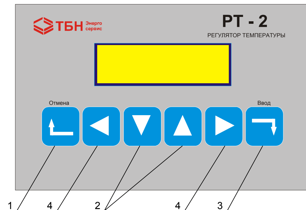
Рисунок 2а. Лицевая панель РТ-2 в раздельном исполнении.
