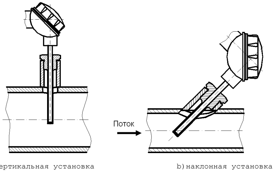
Рисунок П 4.1. Вертикальная и наклонная установка термометров.
