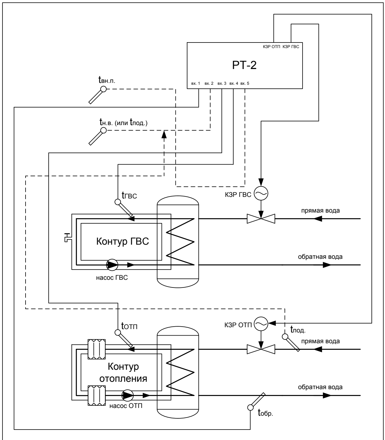
Рисунок П 3.8. Схема подключения регулятора РТ-2 при использовании на ЦТП (ИТП) для регулирования системы ОТП и системы ГВС.
