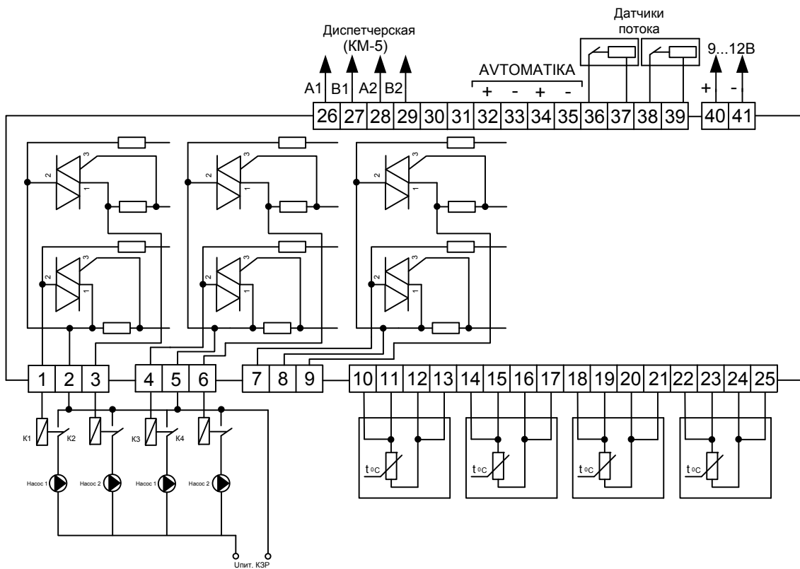
Рисунок П 1.2. Схема подключения насосов и датчиков потока.
