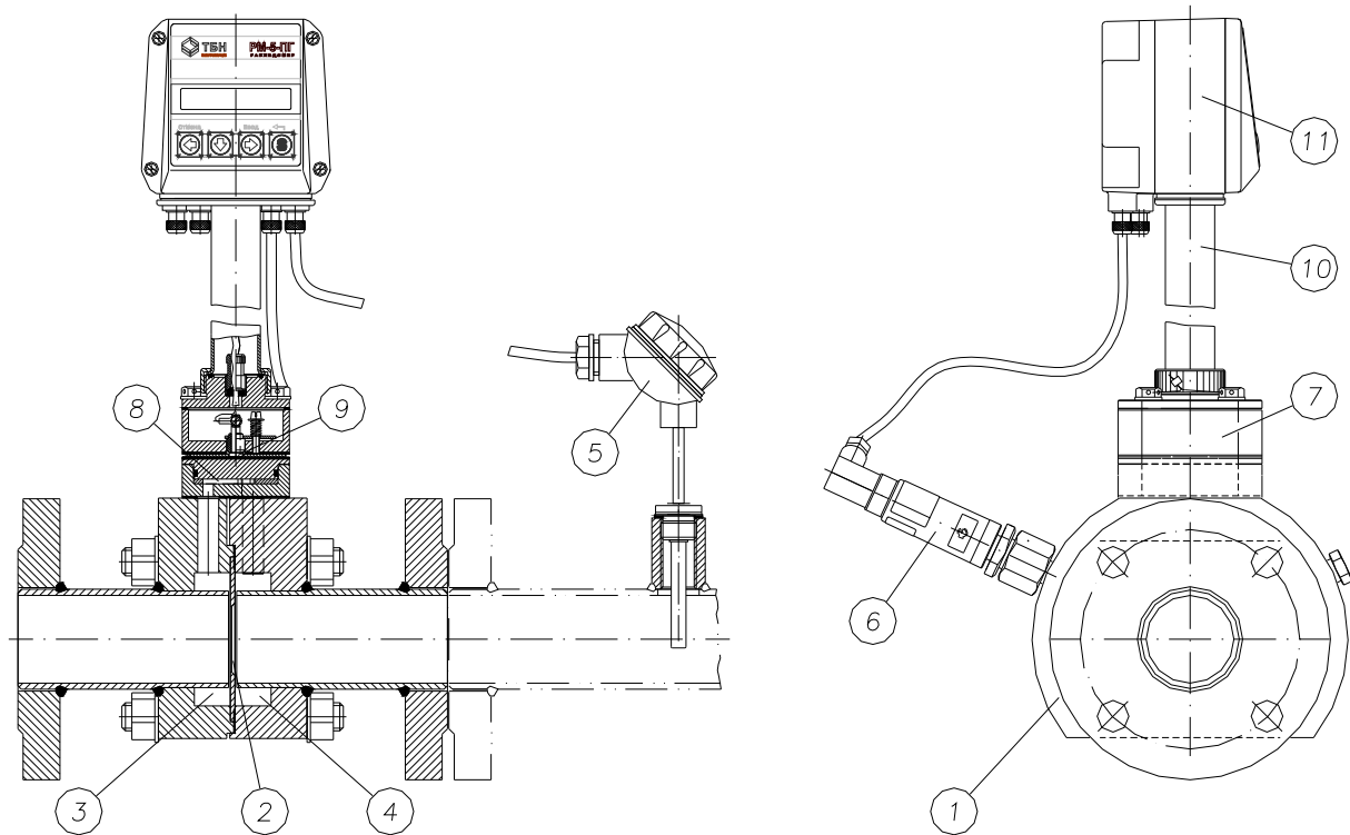
Рисунок 1 Состав расходомера: 1-СУ; 2-диафрагма; 3-КВД; 4-КНД; 5-ПТ; 6-ПД; 7-САГ; 8-струйный элемент; 9-пьезодатчики; 10 – стойка, 11-ЭБ.
