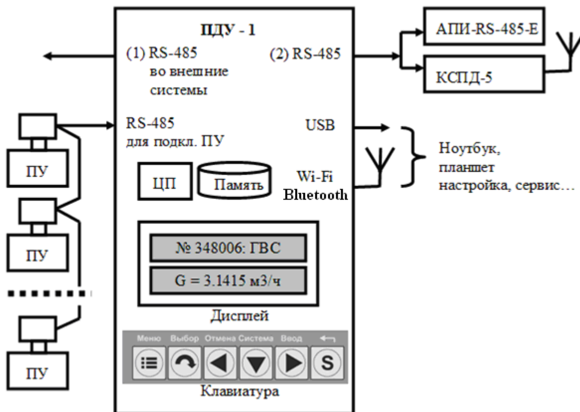
Рисунок 1 — Подключение ПДУ-1 к приборам учёта, компьютеру и внешним системам
