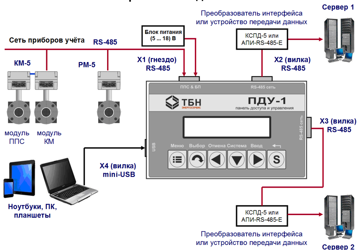
Рисунок А.1 — Состав и назначение разъёмов ПДУ-1
