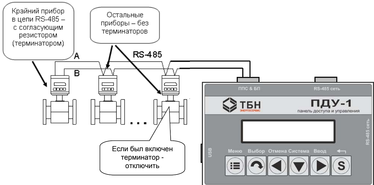
Рисунок 3— Подключение к сети RS-485
